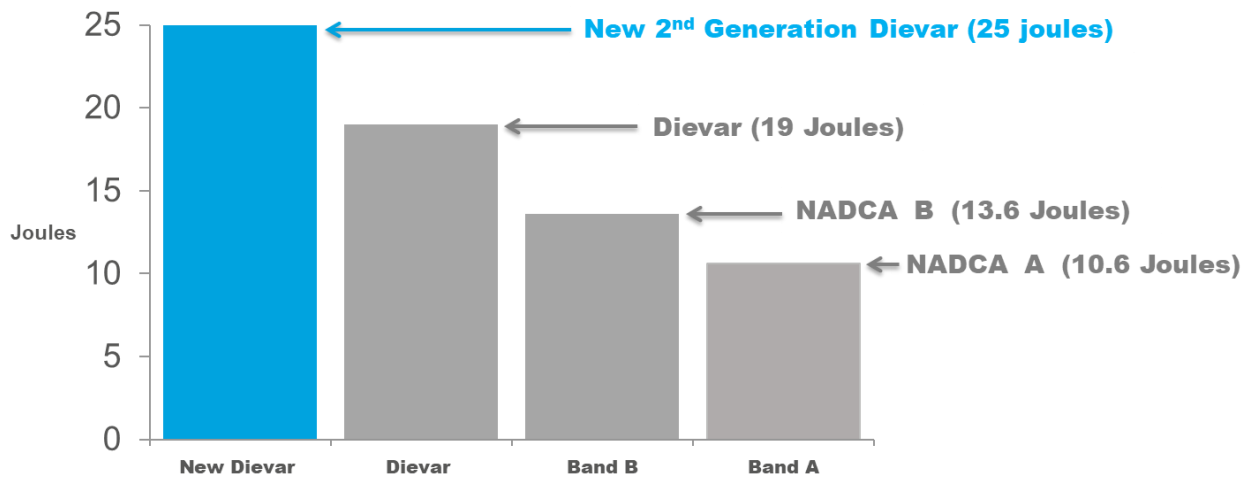
La imagen 1 muestra el aumento de tenacidad del nuevo Uddeholm Dievar
