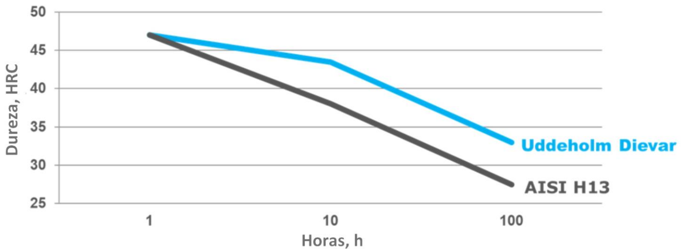
La Figura 7 ilustra una de las múltiples ventajas de la composición química de Uddeholm Dievar sobre H13 para hacer frente al choque térmico y resistencia superior ante la pérdida de dureza
