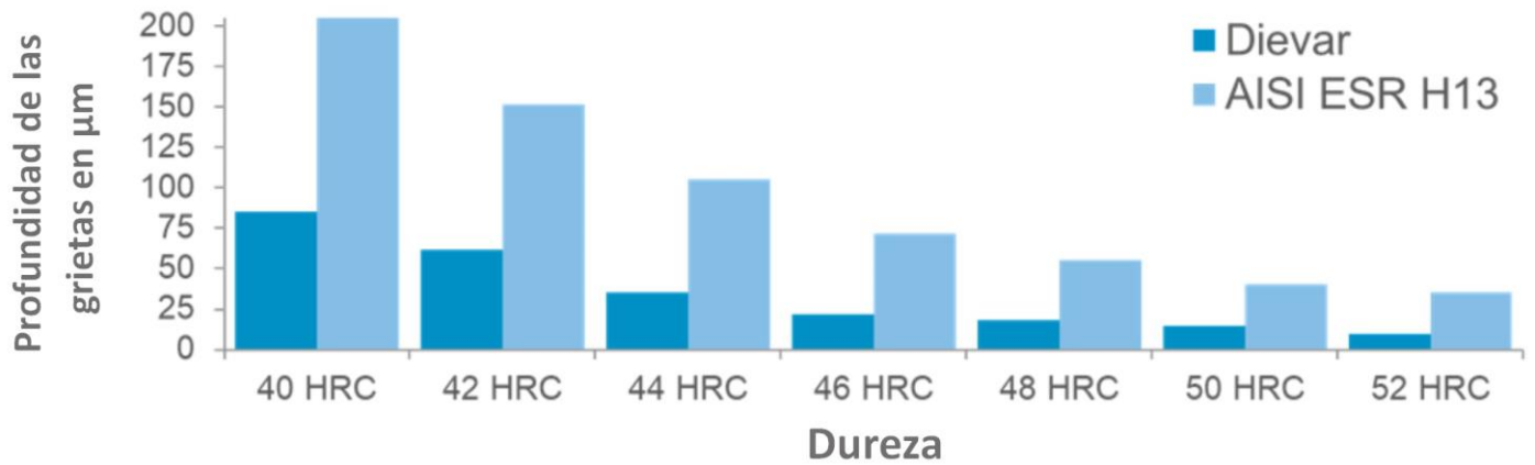
La imagen 5 ilustra como Uddeholm Dievar presenta mayor resistencia ante el agrietamiento por choque térmico que el acero premium H13
