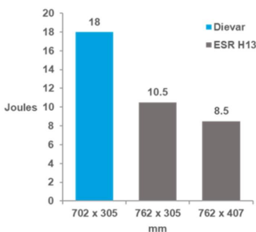
La Imagen 6 muestra como Uddeholm Dievar con mayor dureza también es más tenaz que el acero premium H13
