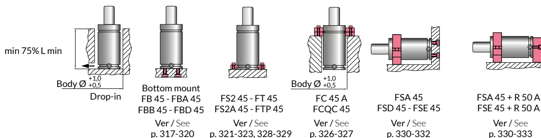
Recomendación de montaje / Assembly recommendation
