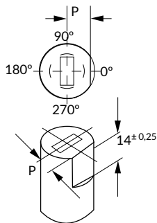
AG 5 Fresado arriba Step flat top
