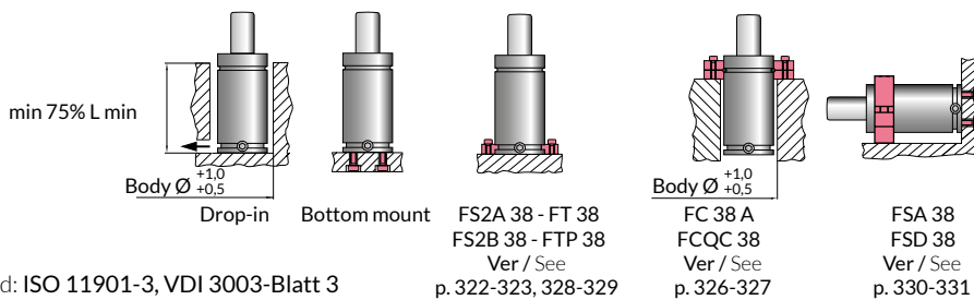
Recomendación de montaje / Assembly recommendation
