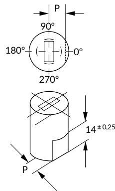
AG 6 Fresado abajo Step flat bottom
