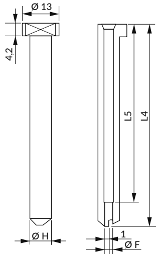
Punzón de embutición / Drawing punch
