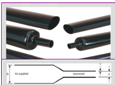
Tubo termoretráctil de pared media y gruesa
