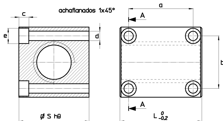
Sección A-A
