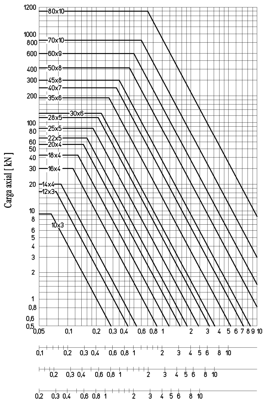
Gráfico n° 6: Carga límite
