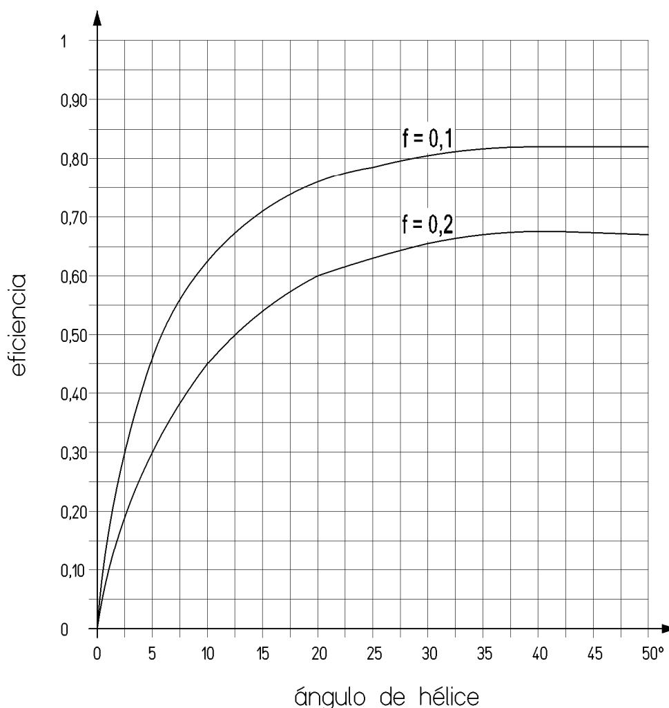
Gráfico n° 8: Eficiencia
