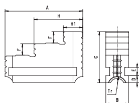
Garras duras monoblock
