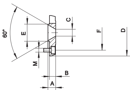
Tope para centro de fuerza elástico-mecánica
