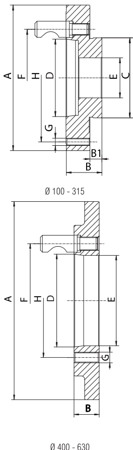
DIN 55029 - Tipo 8245
