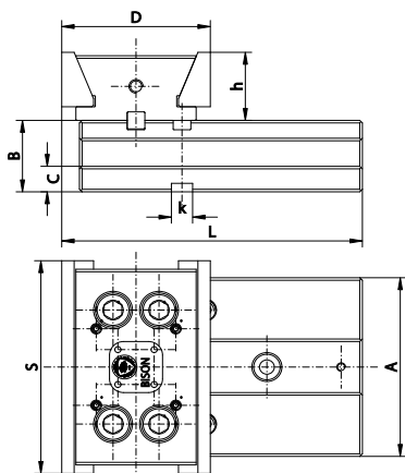
Elemento fijo de doble boca trasera
