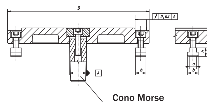
Cono Morse
