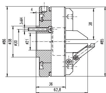
3868 ø85
