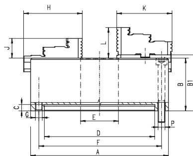
Plato universal amarre frontal Tipo 3274, 3275, 3574, 3575
