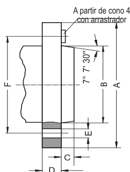
DIN 55027 & ISO 702/III
