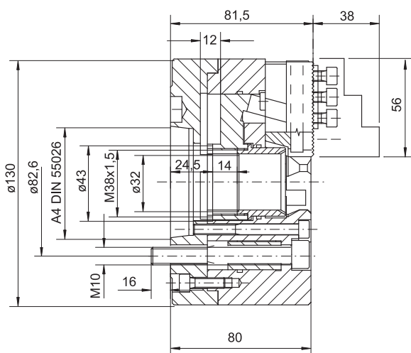
Tipo 2409-130A4
