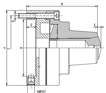
Pinza de sujeción 5C (no incluido)
