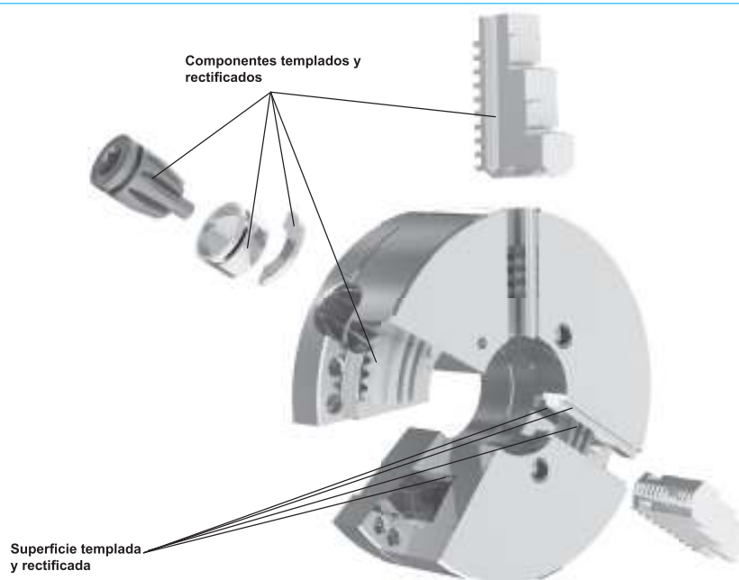
Platos tipo 3500, 3700
