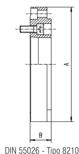
DIN 55026 - Tipo 8210
