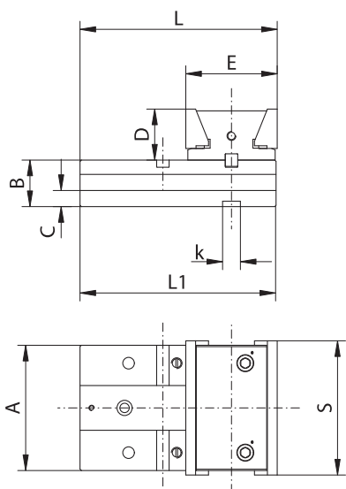
Elemento fijo de doble boca trasera
