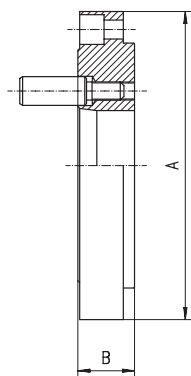
DIN 55029 - Tipo 8240
