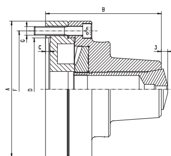
Pinza de sujeción 5C (no incluido)
