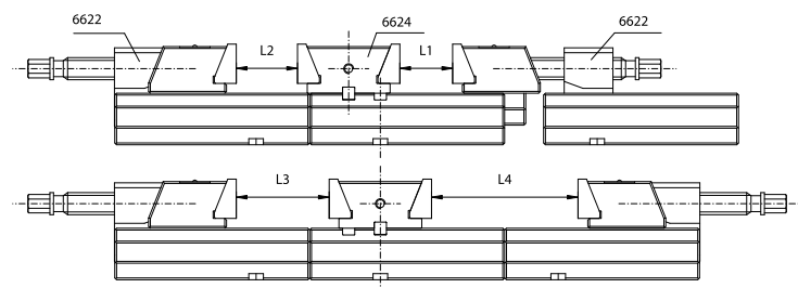
Elemento fijo de doble boca trasera
