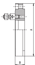
DIN 55027 - Tipo 8230
