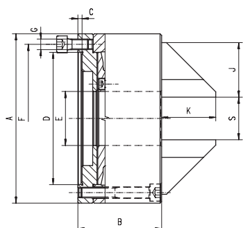
3867 ø160
