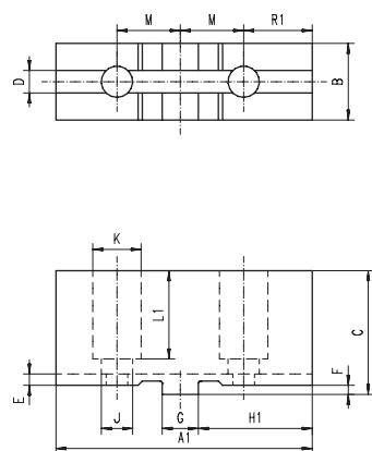
Garras blandas postizas
