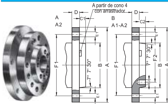
DIN 55026 Tipo A Tipo B - ISO 702/I Tipo A2 Tipo A1-A2
