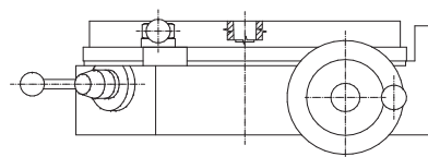
Uso del adaptador tipo 8293
