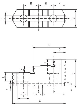
Garras duras postizas reversibles
