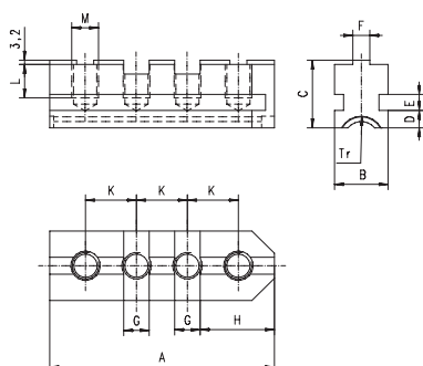
Garras duras base
