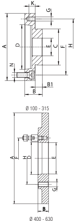
DIN 55029 - Tipo 8245
