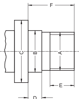
DIN 800
