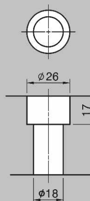
M16 沉頭孔
