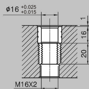
φ16 定位螺絲孔
