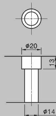
M12 沉頭孔
