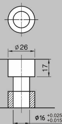
M16 定位沉頭孔
