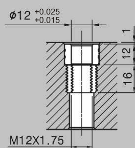
φ12 定位螺絲孔
