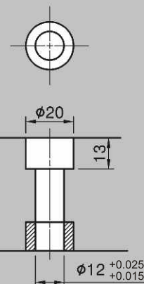
M12 定位沉頭孔
