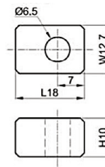
Estación E Superior mod.2 Station E Upper Key mod.2
