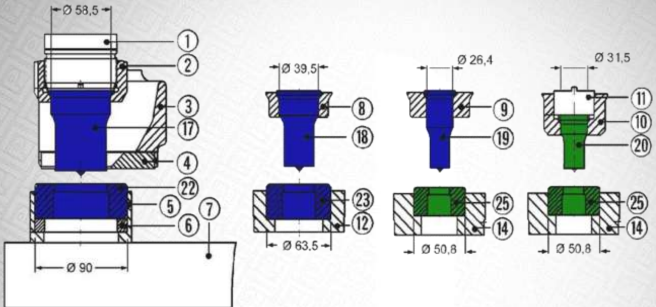
Portamatriz universal Para ángulos y perfiles
